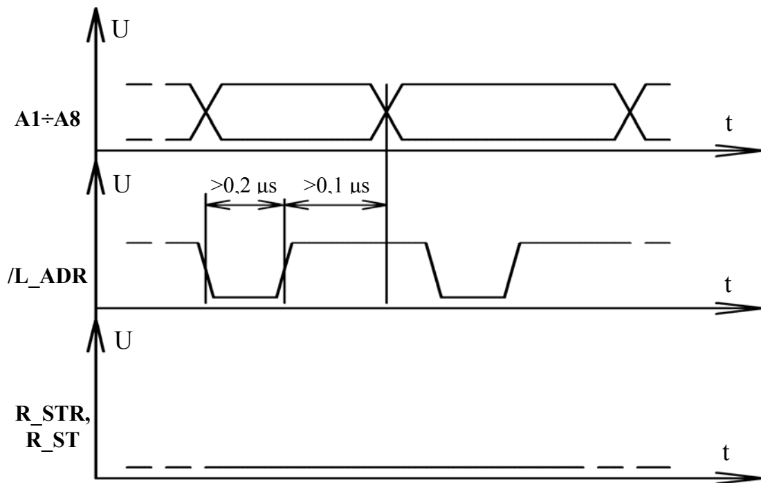
Рис 1. Запись адреса знакоместа в адресный счетчик
